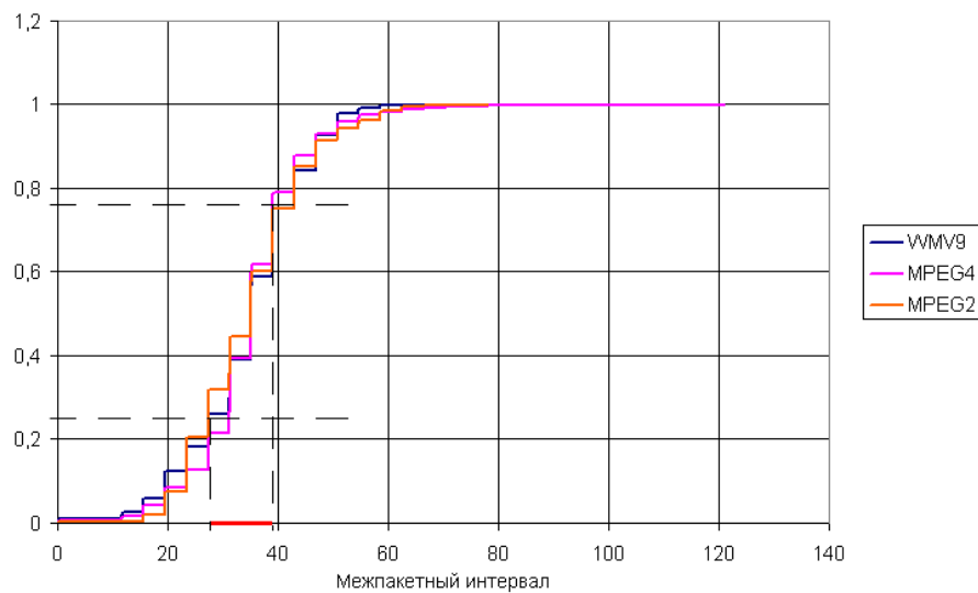
Рисунок 2 Функция распределения межпакетного интервала исходного потока
